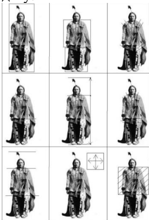
Рисунок 1 – Системно-структурний аналіз
