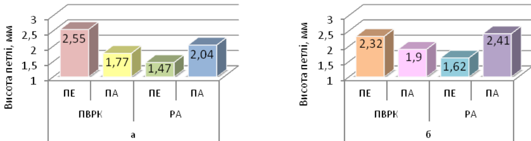
Рис. 6. Діаграми висоти петлі дослідних зразків трикотажу з поліетиленової та параарамідної ниток: а – без металеві мононитки, б – з металеві монониткою
