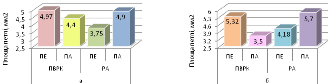
Рис. 7. Діаграми площі петлі дослідних зразків трикотажу з поліетиленової та параарамідної ниток: а – без металеві мононитки, б – з металеві монониткою
