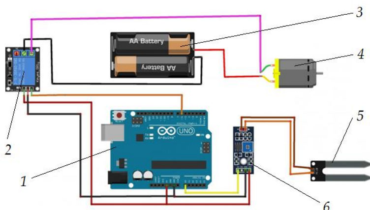
Рис. 2. Схема автоматизованої системи поливу на основі Arduino: 1 – керуючий пристрій (Arduino); 2 – реле, що вмикає насос; 3 – блок живлення; 4 – насос; 5 – датчик вологості ґрунту; 6 – електронна плата датчика вологості
