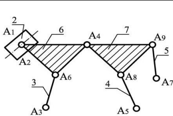
Рисунок 1 – Структурна група третього класу четвертого порядку з восьми обертальними та однією поступальними кінематичними парами
