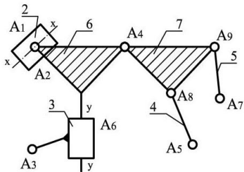
Рисунок 2 – Структурна група третього класу четвертого порядку з восьми обертальними та двома поступальними кінематичними парами
