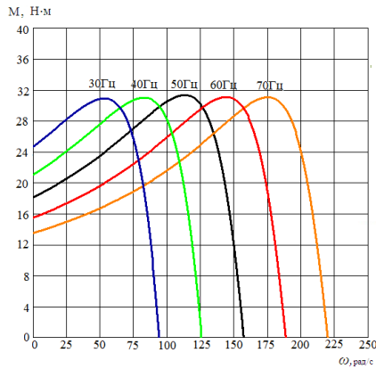
Рис. 8. Механічні характеристики електродвигуна 4А50В2У3 з синхронною частотою обертання 3000 об/хв при різних частотах живлення за законом керування U_{\phi} / f = const
