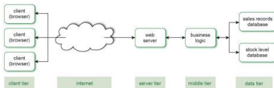
Рисунок 2.2- Рисунок 2.2 Схема багаторівневої архітектури
