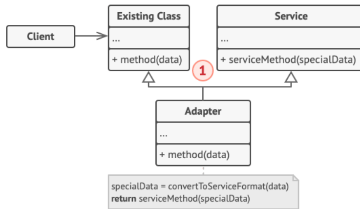
Рисунок 1.7 - Структура адаптера класів
