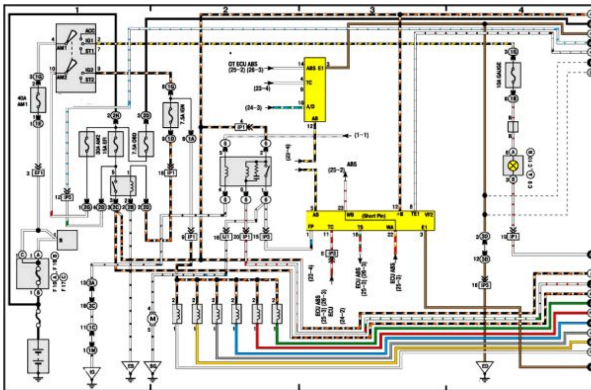
Рис. 1. Електрична схема керування двигуном автомобіля Тойота Камрі.
