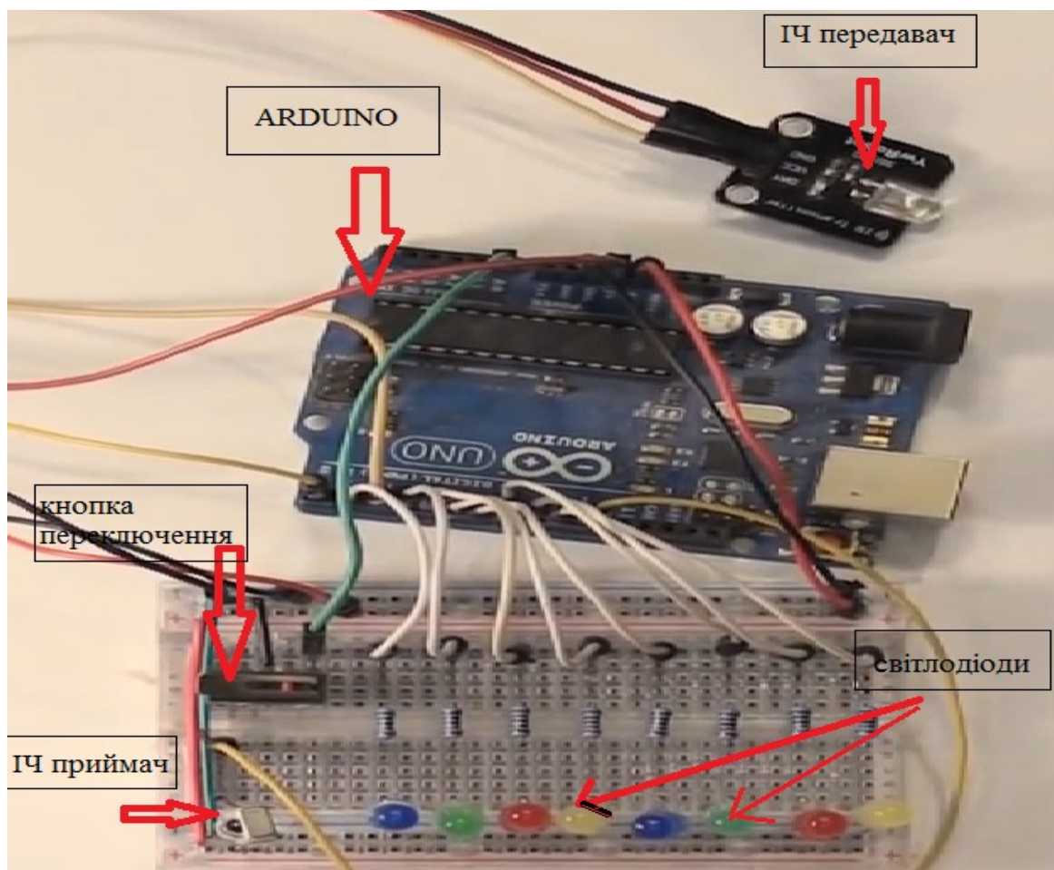
Рис.1. Вид «універсального» пульта на платформі ARDUINO
