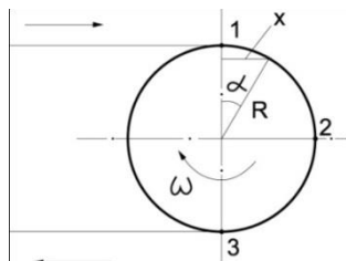
Рис. 1. Траєкторія руху пальця повзуна проміжної каретки рукавичного автомату на криволінійній ділянці траси ланцюга
