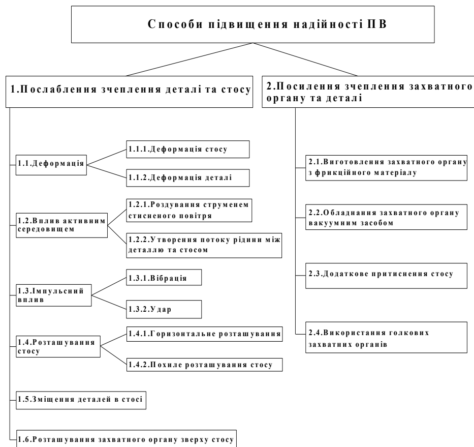
Рисунок – Способи покращення умов процесу поштучного відокремлення
