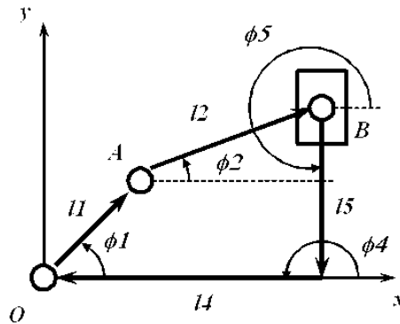
Рис.1. Кінематична схема
