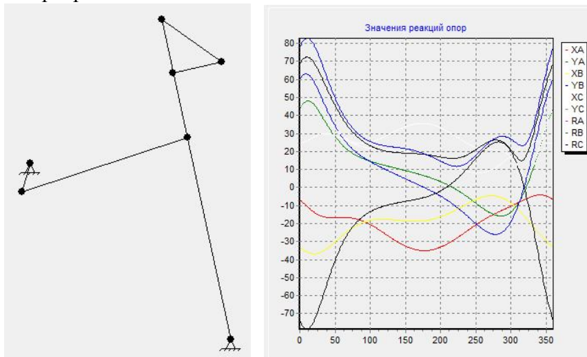
Рисунок 1 – Схема батанного механізму верстата типа АМВ та основна форма програми
