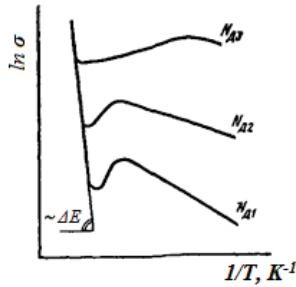
Рис. 3.3. Температурні залежності питомої провідності напівпровідника при різних концентраціях домішок: N_{D1} < N_{D2} < N_{D3} .
