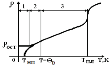
Рис. 2.1. Залежність питомого опору металевого провідника від температури. T_{\text{нп}} – температура переходу у надпровідний стан, T_{\text{пл}} – температура плавлення
