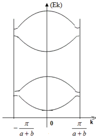
Рис. 1.12. Перша зона Бріллюена.
