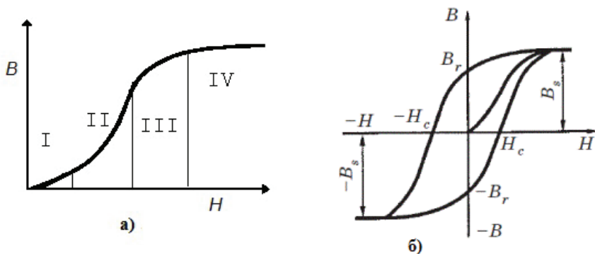
Рис. 5.1. Крива намагнічення а) і петля гістерезису б).
