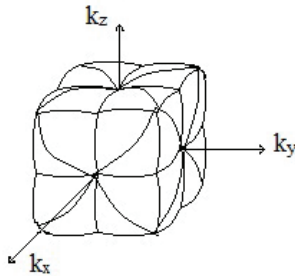
Рис. 1.14. Ізоенергетичні поверхні в k просторі біля стелі важких дірок в валентній зоні кремнію та германію.
