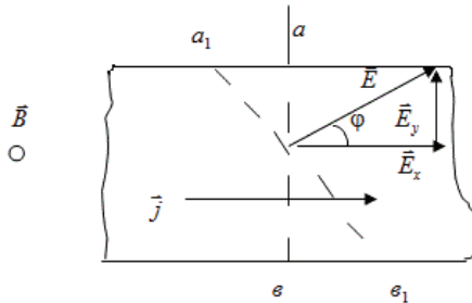
Рис. 3.5. Схема утворення поля Холла \vec{E}_y .
