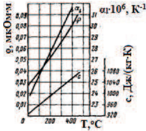
Рис. 2.4. Залежності питомого опору \rho , питомої теплоємності c та температурного коефіцієнта лінійного розширення \alpha_l від температури для алюмінію.
