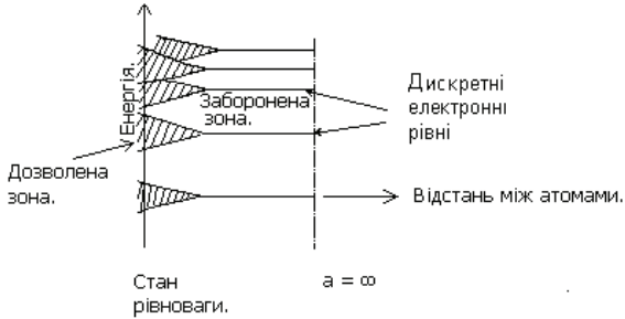
Рис.1.9. Схема утворення енергетичних зон.
