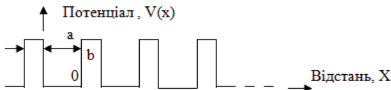
Рис. 1.10. Прямокутний одномірний періодичний потенціал.
