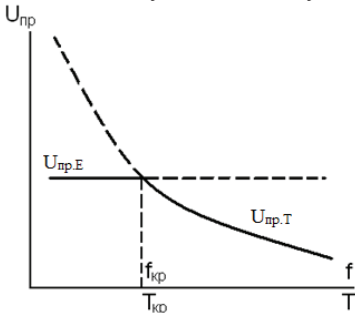
Рис. 4.4. Типова залежність пробивної напруги від частоти і температури.
