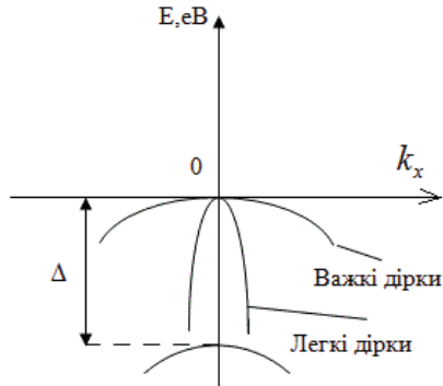
Рис. 1.15. Валентна зона кремнію. Енергетичні зони.
