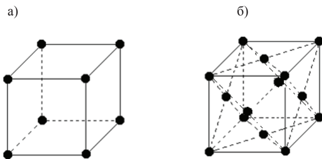
Рис. 1.6. Гратки Браве – проста кубічна (а) і гранецентрована кубічна (б).
