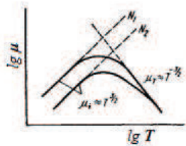
Рис. 3.4. Температурна залежність рухливості носіїв заряду для невиродженого напівпровідника при різних концентраціях домішок.
