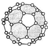
Рис. 2.6. Фулерен
