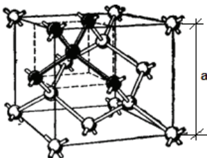
Рис.1.3. Модель кристалічної ґратки алмазу.
