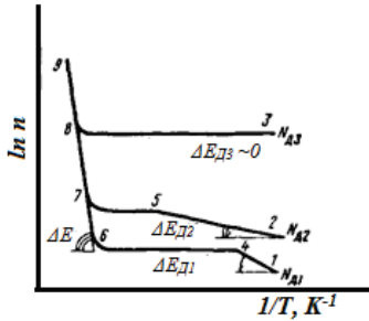
Рис. 3.1. Характерні залежності концентрації носіїв заряду в напівпровіднику від температури при різних концентраціях донорних домішок N_{Д1} < N_{Д2} < N_{Д3}
