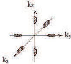
Рис. 1.13. Ізоенергетичні поверхні зони провідності кремнію.
